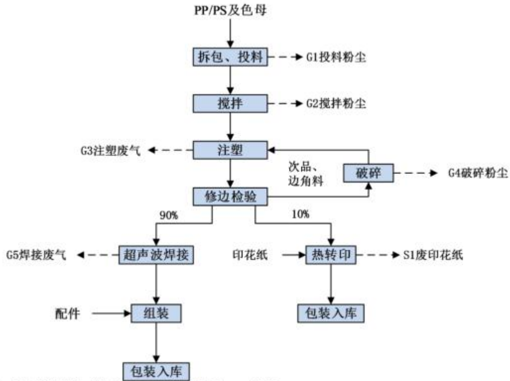
图 2-1 项目生产工艺流程及产污节点图
